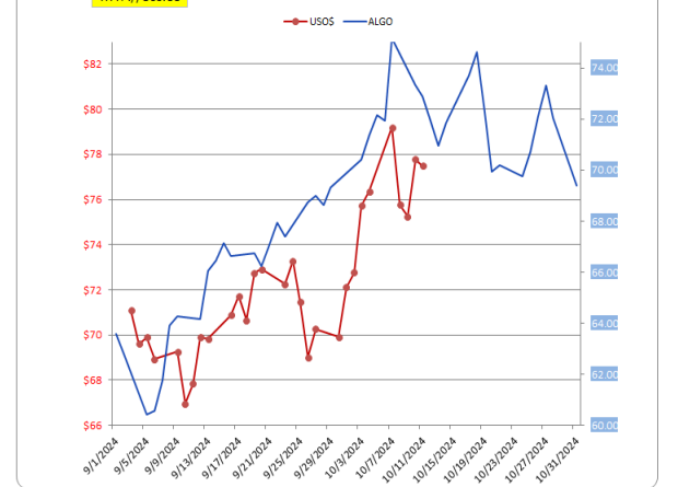
ALGO Forecast vs USO
